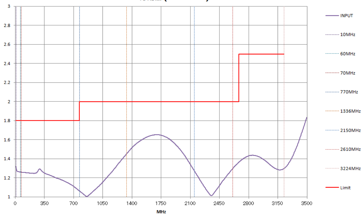
VSWR(IN) 3.2GHz 2分配器 (SPJ-2K8A)
