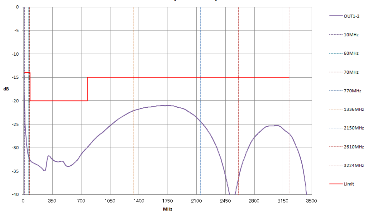
端子間結合損失(OUT 1-OUT 2) 3.2GHz 2分配器 (SPJ-2K8A)
